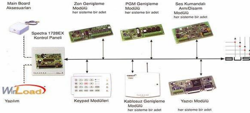
Şekil 1.3: Soygun alarm sistemlerinde kullanılan devreler ve bağlantılar
